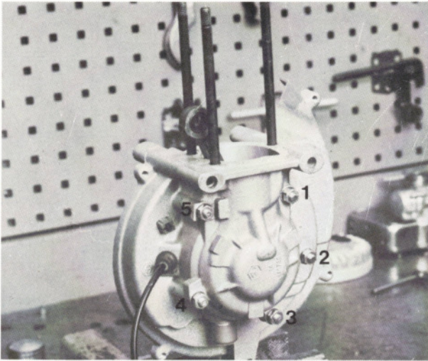
Befestigungsschrauben (1-5) der Gehäusehälfte abschrauben. (SW 10)
