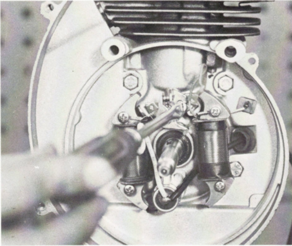
Unterbrecher einsetzen.
