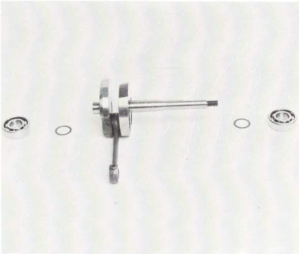
Kurbelwelle mit Lagern und Anlaufscheiben.
