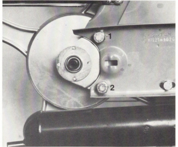
Schraube 1 u. 2 lösen. (SW 17)
