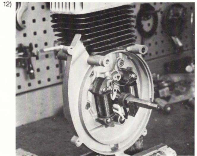
Federscheibe und Nocken abnehmen.
