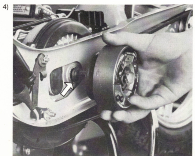
Kupplungskorb herausziehen. Beim Einbau beachten, daß die breite Auflagefläche der Scheibe gegen den Rotor liegt. (Siehe Pfeil)
