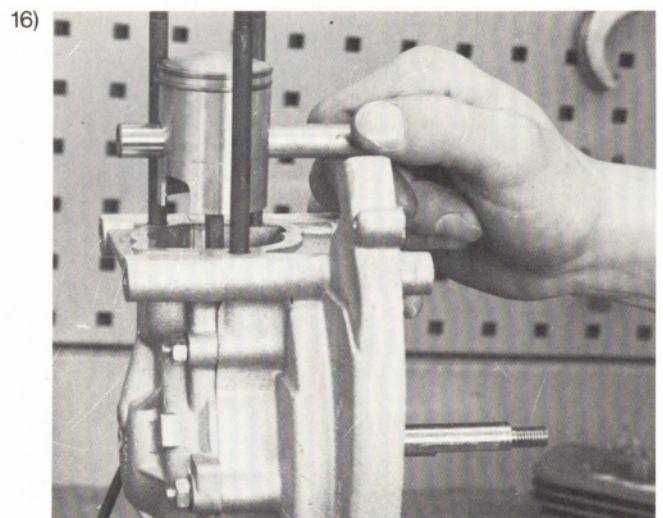
Kolbenbolzen herausdrücken.
