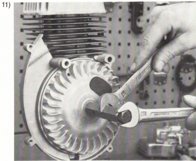
Rotor mit Abzieher T 0035485 abnehmen.
