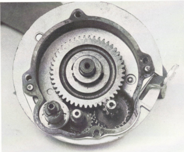
Getriebe in geöffnetem Zustand. (Öl abgelassen)
