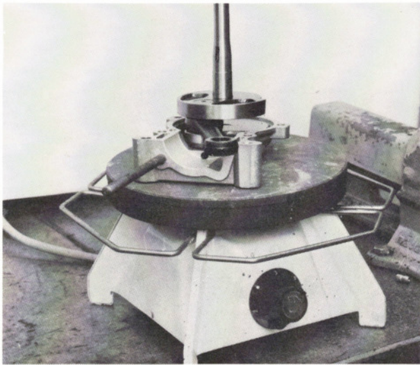
Gehäusehälfte erhitzen und Kurbelwelle von Hand herausziehen.
