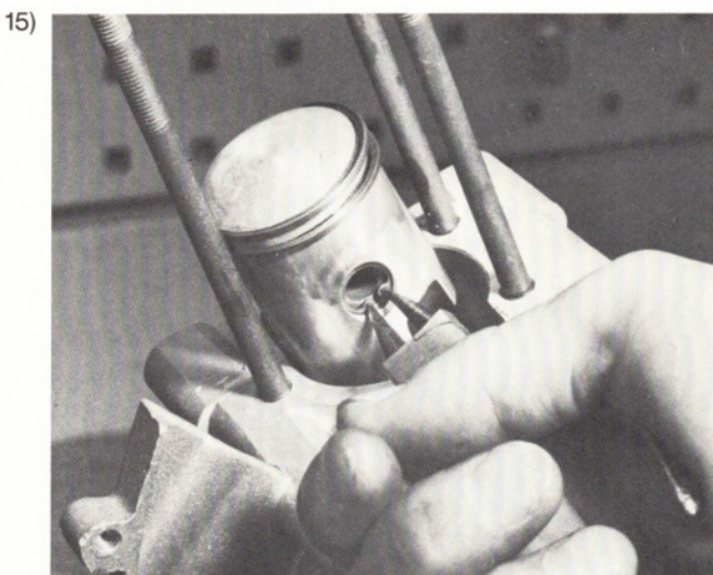
Seegerringe des Kolbenbolzens links u. rechts ausfedern.
