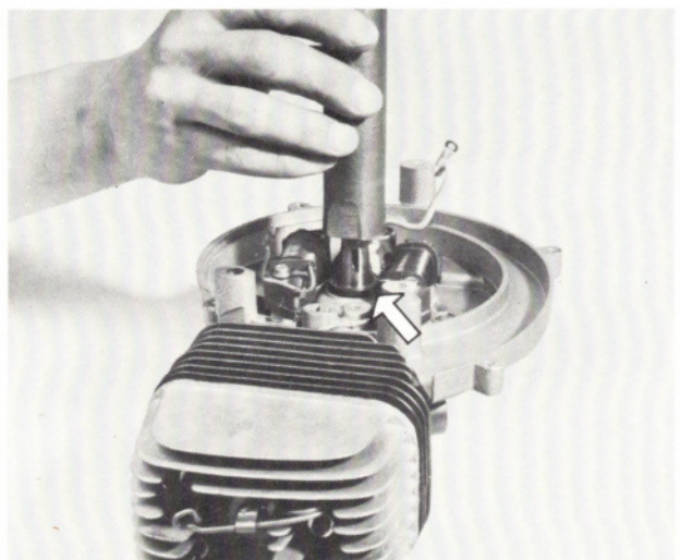
Wellendichtring mit Dorn einsetzen. (s. Pfeil)
