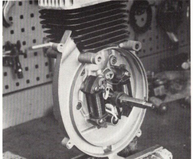
Federscheibe und Nocken aufsetzen.
