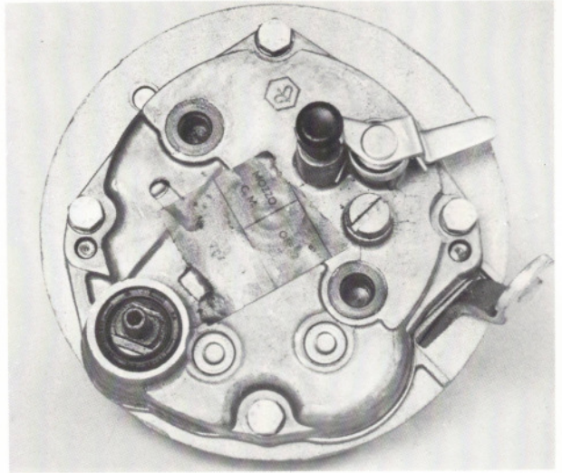
Getriebedeckel abschrauben. (Schrauben 1-4) (SW 10)
