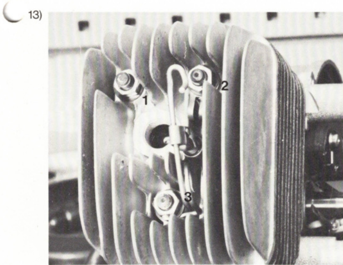
Muttern (1-3) der Zylinderkopfbefestigung lösen. (SW 11)
