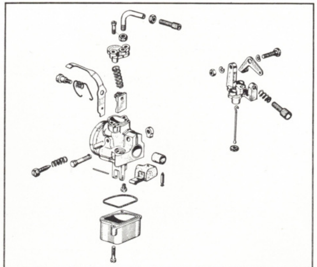
Explosions-Darstellung „Vergaser“
