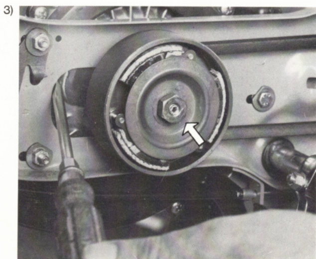
Rotor mit Schraubenzieher blockieren. Mutter des Kupplungskorbes abschrauben. (Siehe Pfeil/SW 13)
