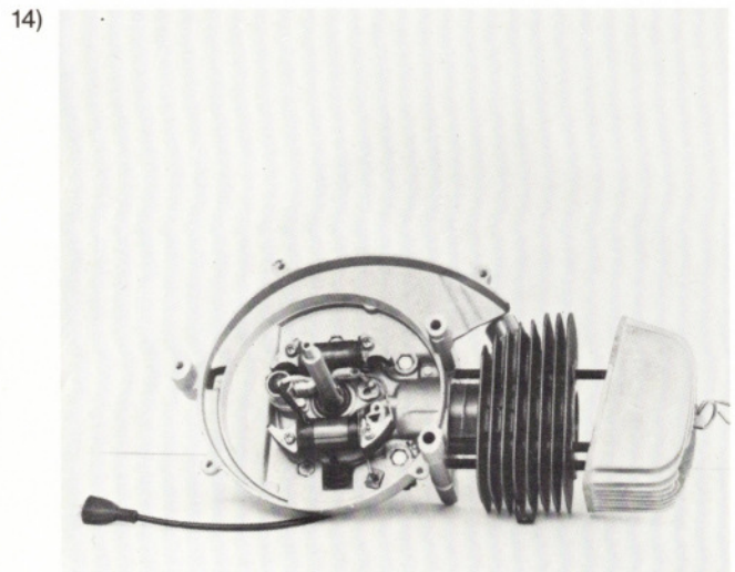
Zylinderkopf und Zylinder abnehmen.
