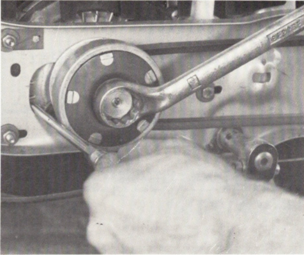
Abnehmen des Wandlers
