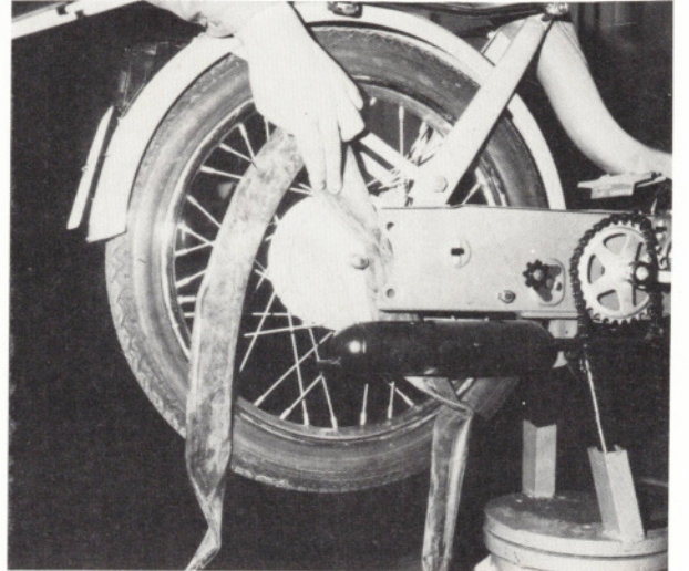
Schlauch zum Auswechseln bzw. Flickern durch die entstandene Öffnung ausfädeln. Das Hinterrad bleibt fest eingebaut.
