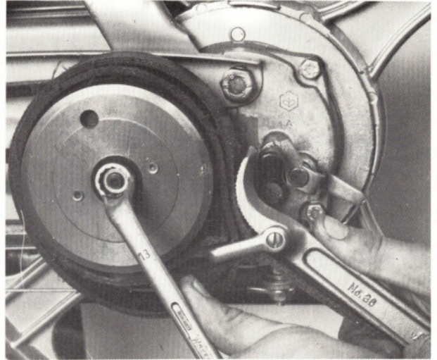
Abnehmen des Kupplungskorbes mit Druckausgleichsfeder.
