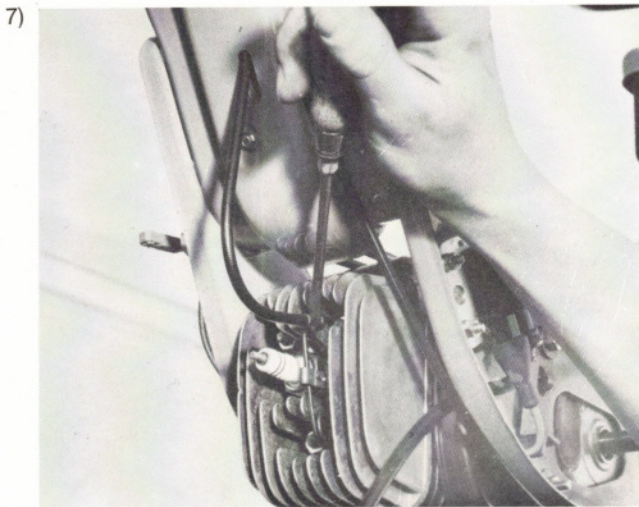
Dekompressionszug aushängen. (Federklammer mit Schraubenzieher nach hinten drücken, Zug aushängen.)
