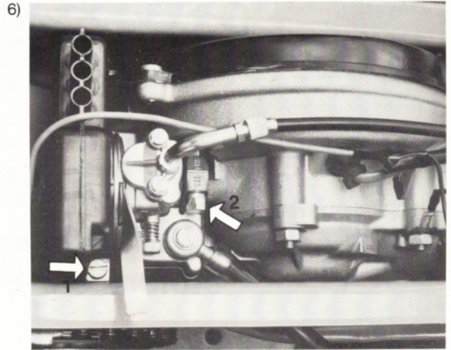
Klemmring am Luftfilter lösen (1) und Luftfilter abnehmen. Klemmring am Vergaser lösen (2) und Vergaser abnehmen. (SW 8)
